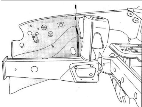
103 – Felicia nosník prahu obj.č.- Lavý 6U5-6-1 / Pr. 6U5-6-2
